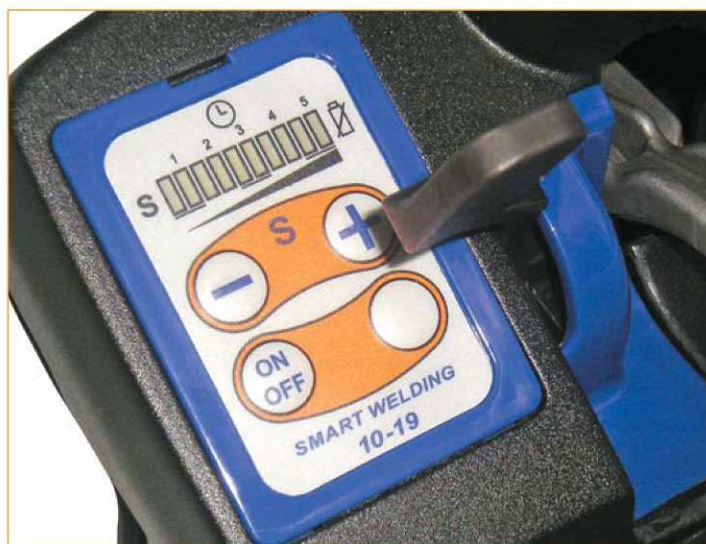
Nuovo sistema tastiera digitale per variare tensione e tempo di saldatura
